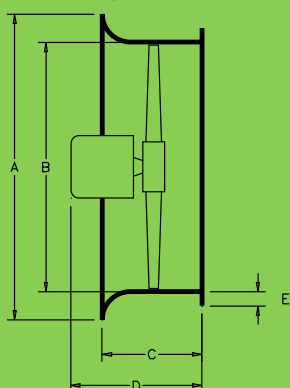
Поперечное сечение вентилятора
